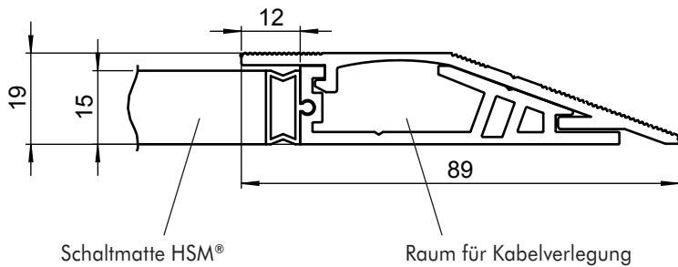
Alu-Rampenprofil (R 2)
