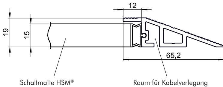
Alu-Rampenprofil (R 1)
